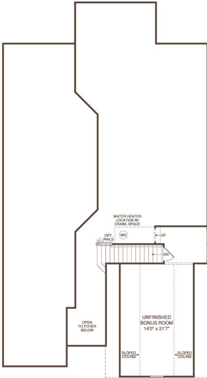
Elevation E
